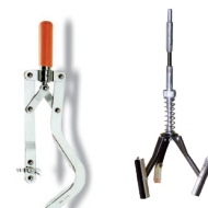
Dụng cụ cạo muối rãnh xéc măng
