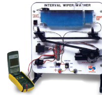
Module đào tạo hệ thống gạt mưa SGN - T11
