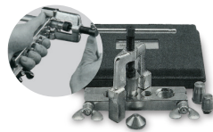
Thiết bị cắt và lọc ống điều hòa
