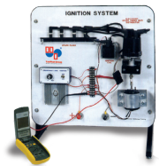
Module đào tạo hệ thống đánh lửa SDLBD-T11
