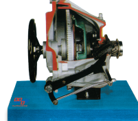
Mô hình cắt bỏ ly hợp ma sát VSCCD - H01
