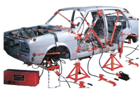
Bộ kéo nắn vỏ xe loại xách tay
