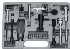
Bộ dụng cụ điều chỉnh nhiên liệu
