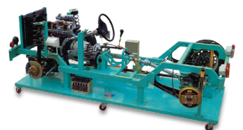
Mô hình cắt bỏ ô tô OTOD44 - H11
