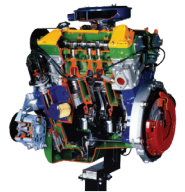
Mô hình cắt bỏ động cơ xăng DX41 - H01
