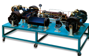
Mô hình hệ thống phanh hơi SPKN4 - H01
