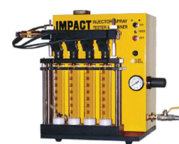
TB kt và làm sạch kim phun
