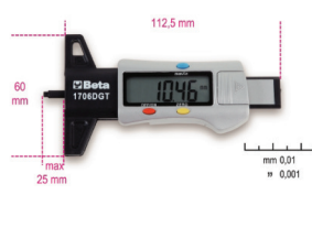
TB Kiểm tra độ sâu hoa lốp hiển thị số
