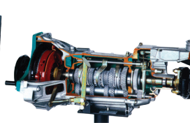
Mô hình hộp số cơ khí HSTDN - T01
