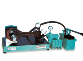
TB kiểm tra và kéo nắn tay biên
